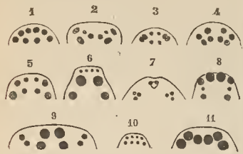
Fig. 1. Disposición de los ojos en las diversas especies de arañas. - 1. Argironeta . - 2. Tenuia . - 3. Teridid . - 4. Aegleona . - 5. Tomito . - 6. Licosa . - 7. Especie afín de las arañas . - 8. Saltador . - 9. Epeira . - 10. Tetragnata . - 11. Segestria .
